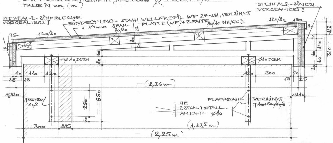
Bau-Zeichnung des neuen Geräteschuppens
